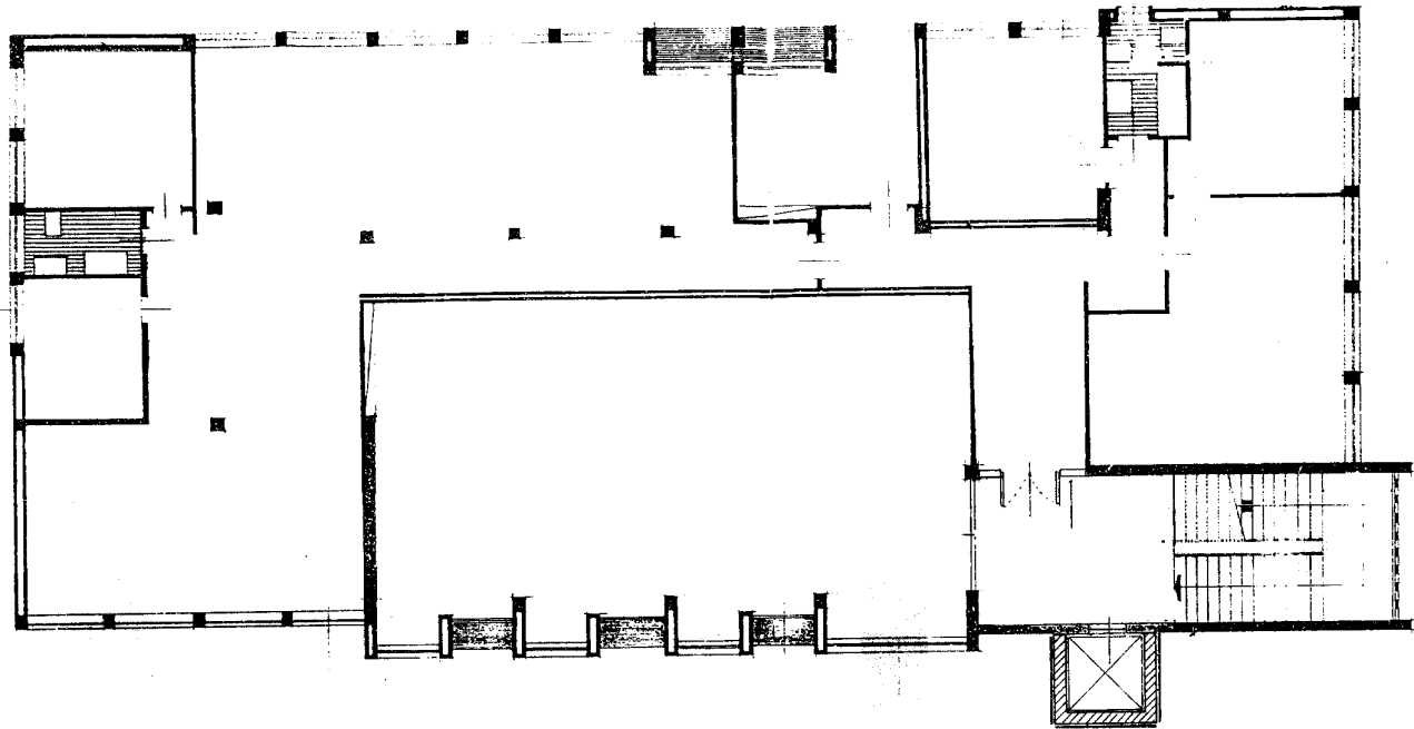
PIANO PRIMO
