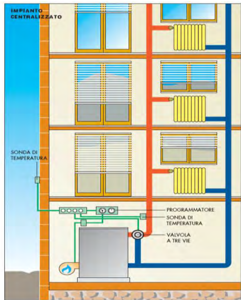
Schema di un sistema di distribuzione
