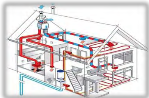
Schema di un impianto di ventilazione
